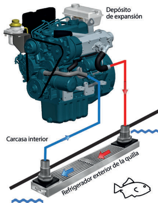
Principio del sistema de refrigeración por quilla en el motor
