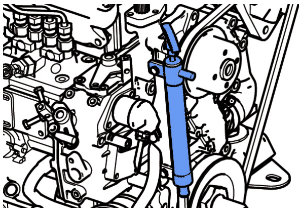
En la imagen superior, la bomba manual (imagen genérica).
