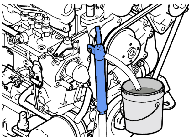
Vista del drenaje de aceite de motor.
