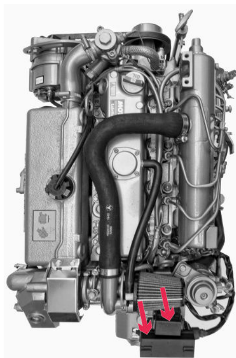
Localización de las cajas de los fusibles y relés
