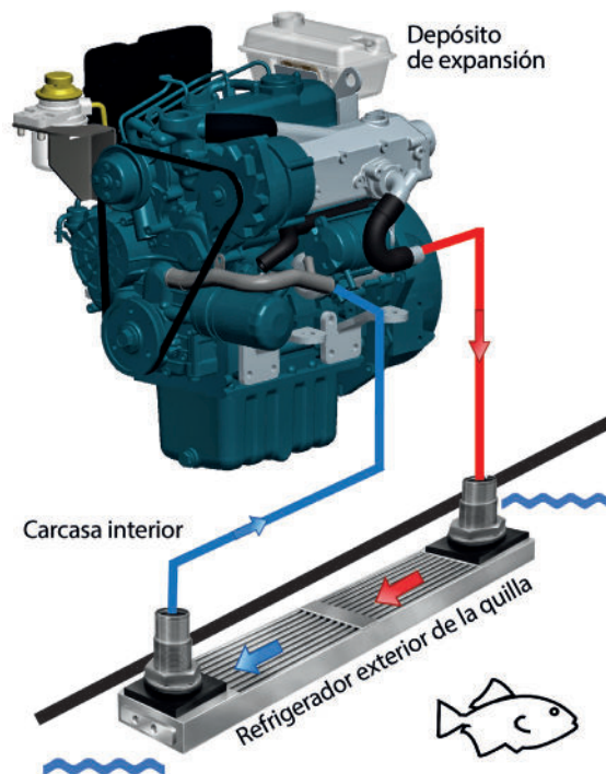
Principio del sistema de refrigeración del motor de quilla
