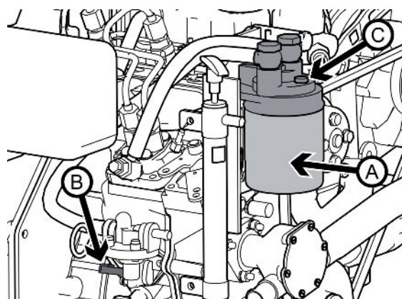
Purga de aire en N2.14 (ventilación C)
