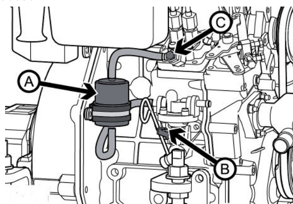
Purga de aire en N2.10 (ventilación C)
