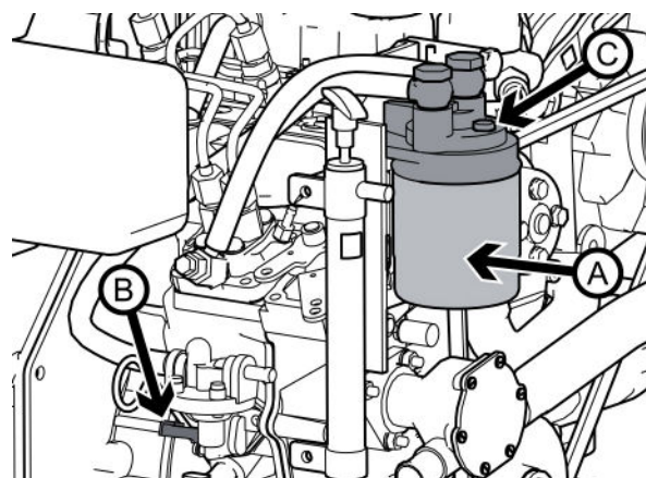
Purga de aire en un N3.21 (válvula C)
