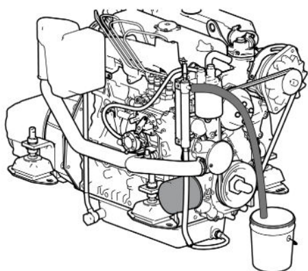
Vista lateral del drenaje de aceite del motor, en la imagen superior.
