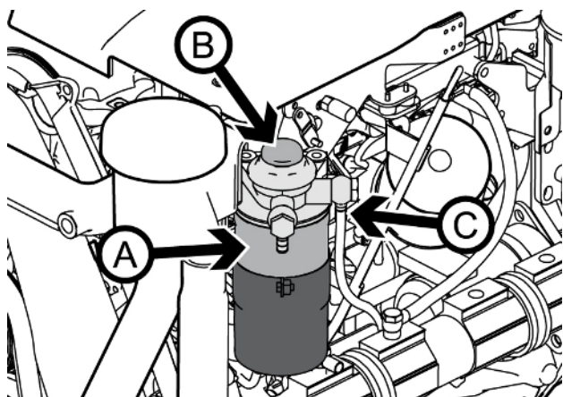
Imagen superior: montaje del filtro de combustible.
