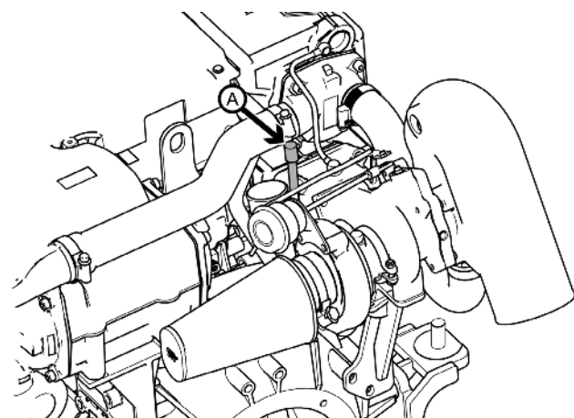
Imagen superior: vista ampliada de la tubería de desagüe.
