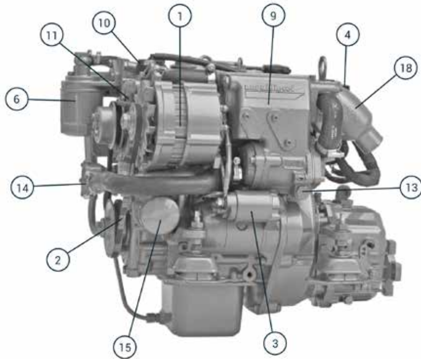
VUES MOTEUR N2.14
