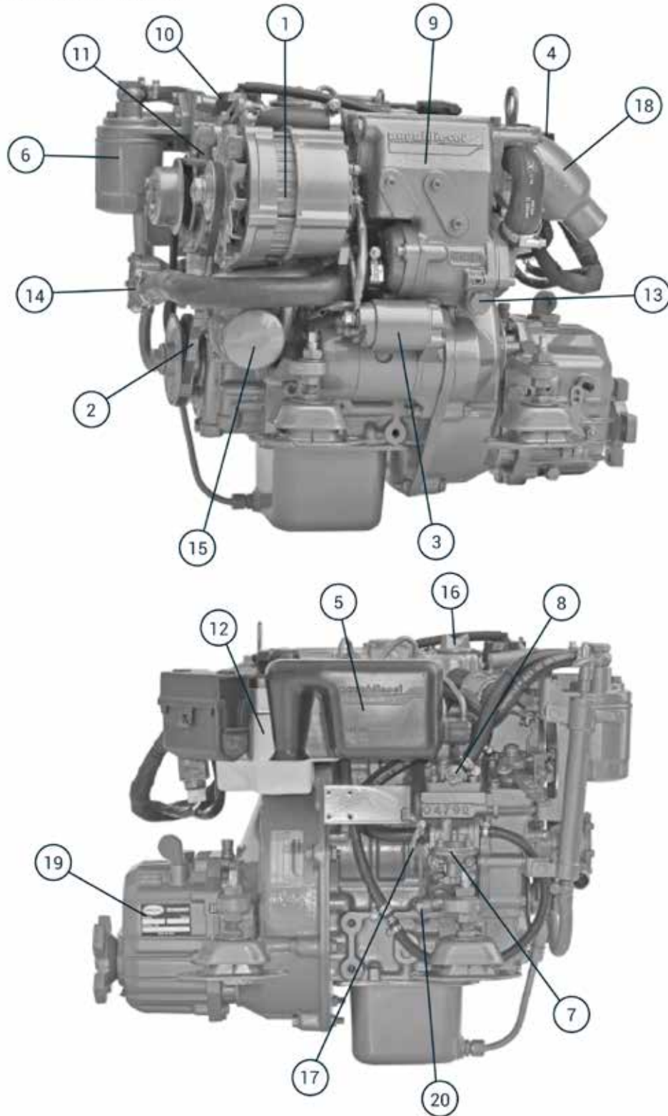
VUES MOTEUR N3.21 - N3.30
