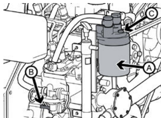
Purge d'air sur le N3.21 - N3.30 (C)
