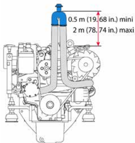
Ci-dessus : l'anti-siphon en bleu.
