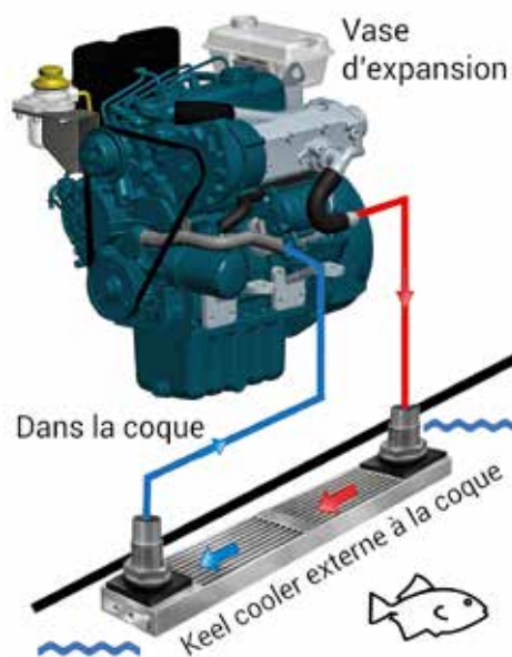
Principe du Keel Cooling
