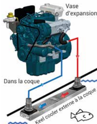
Principe du keel Cooling
