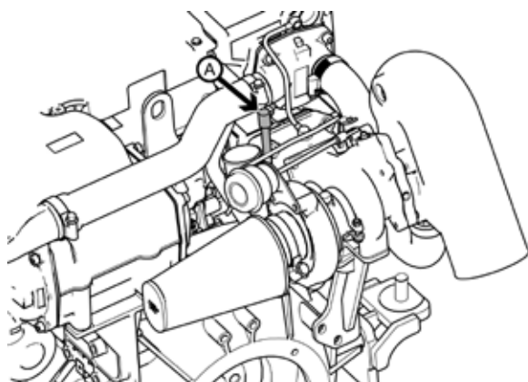
Ci-dessus : dispositif de vidange.
