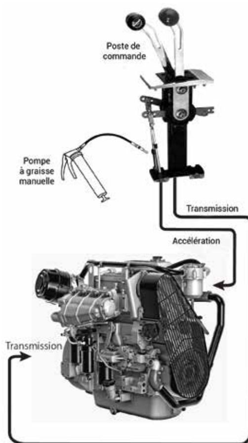
Câbles de commande moteur
