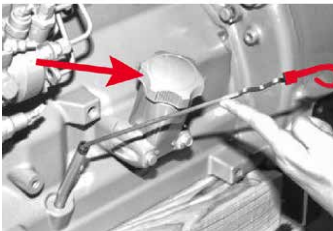
Ci-dessus : ouvrez le bouchon de remplissage d'huile pendant la vidange.
