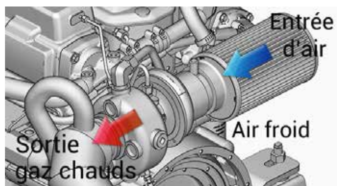
Ci-dessus : Turbo N5 et entrée d'air
