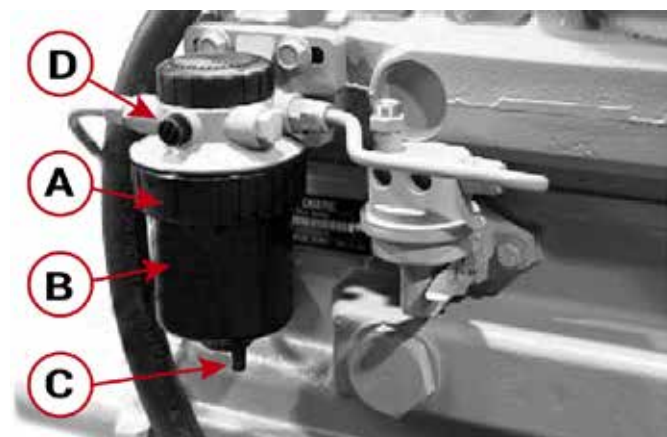
Ci-dessus : l'ensemble filtre à carburant
