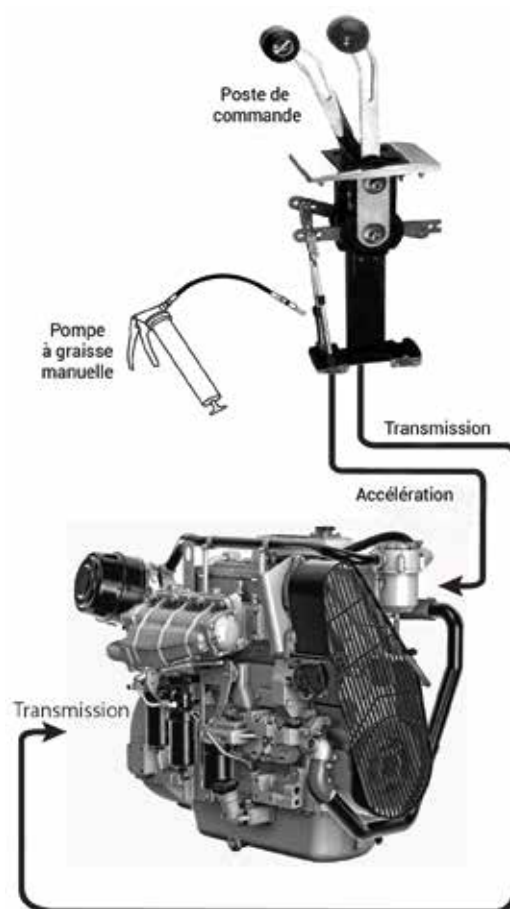
Câbles de commande moteur
