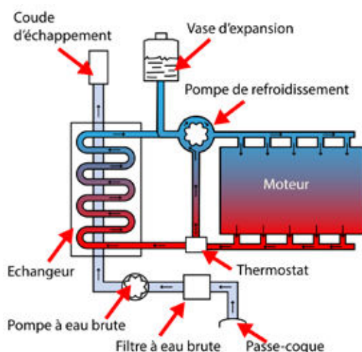
Principe de fonctionnement du refroidissement.
