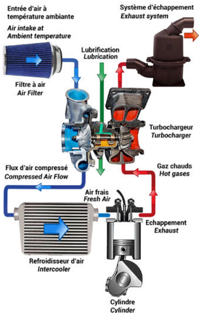
Principe du turbochargeur.
