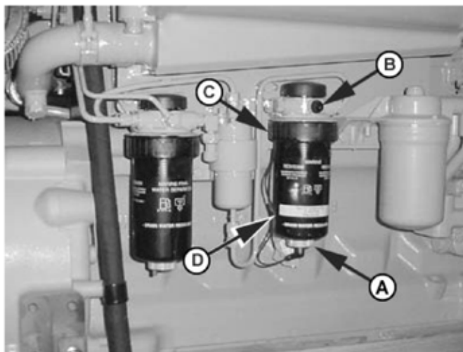
Ci-dessus : le filtre primaire
