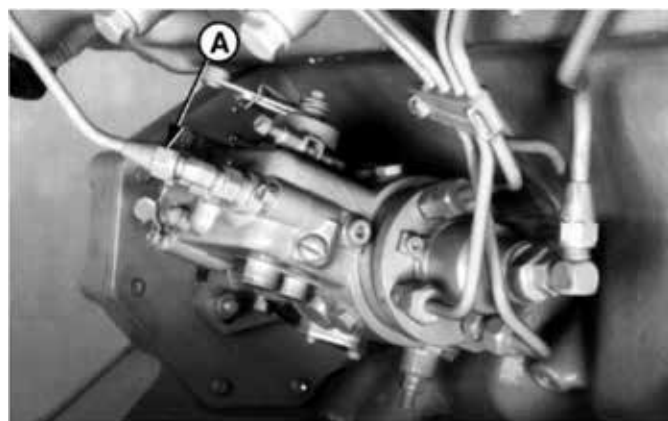
Purge au niveau de la pompe à injection
