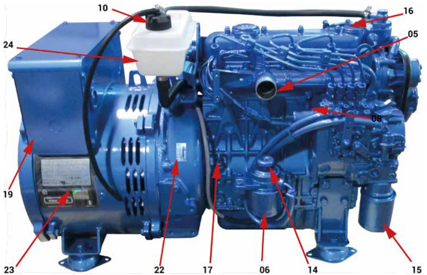
VUE N°2 DU GROUPE ÉLECTROGÈNE
