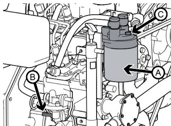
Spurgo dell'aria su N2.14 (sfiato C)
