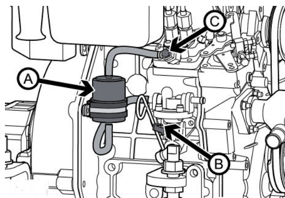
Spurgo dell'aria su N2.10 (sfiato C)
