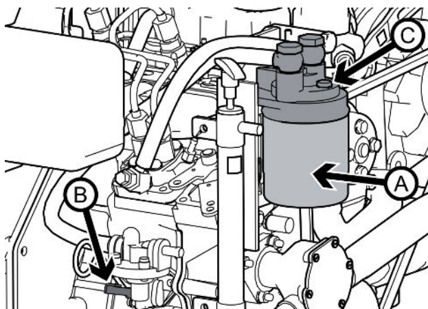
Immagine in alto: rimozione del filtro carburante sul motore N2.14.
