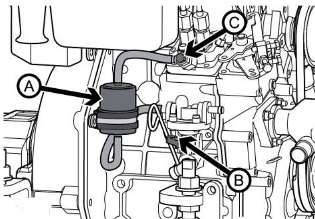
Immagine in alto: rimozione del filtro carburante sul motore N2.10.
