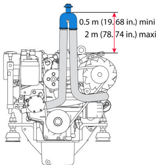
Nell'immagine sopra: rompi-sifone in blu.
