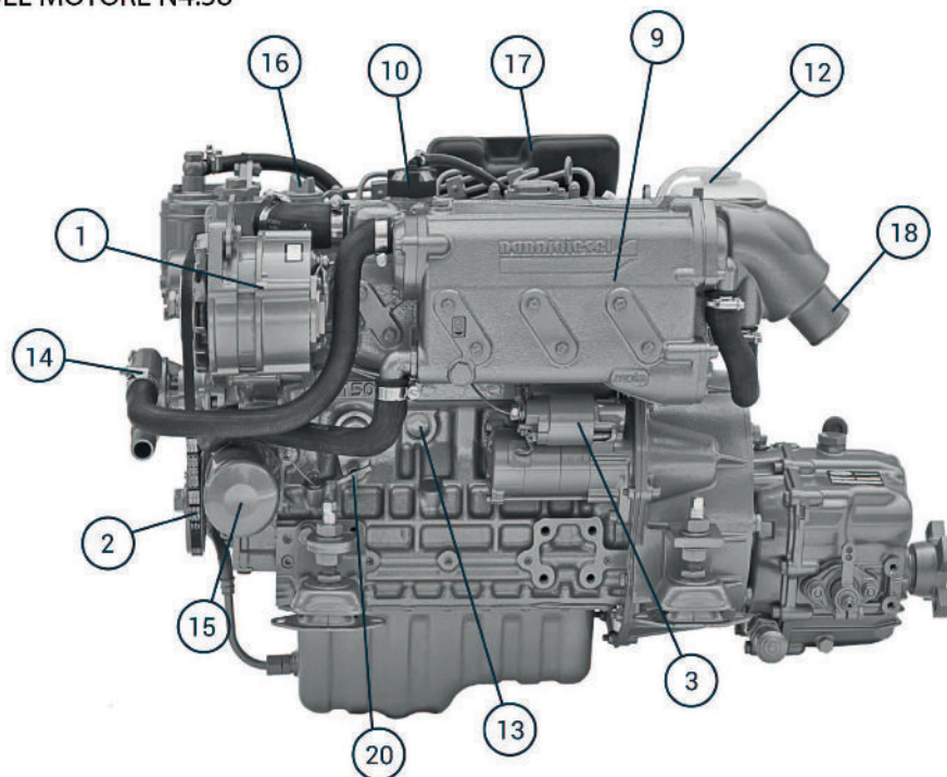
VISUALI DEL MOTORE N4.38
