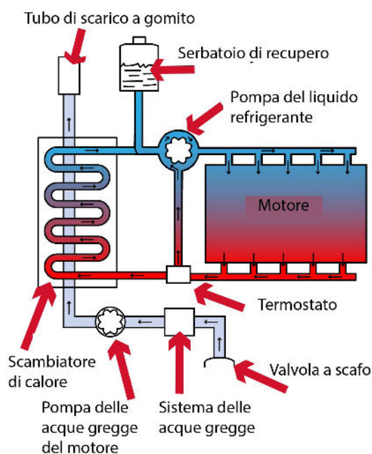
Principio di funzionamento del raffreddamento ad acqua con uno scambiatore di calore sul motore
