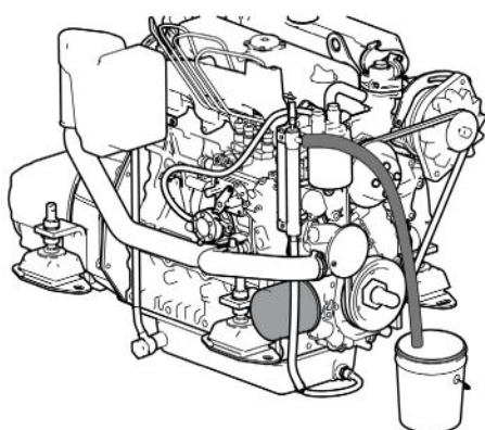
Nell'immagine sopra, visuale laterale del drenaggio dell'olio nel motore
