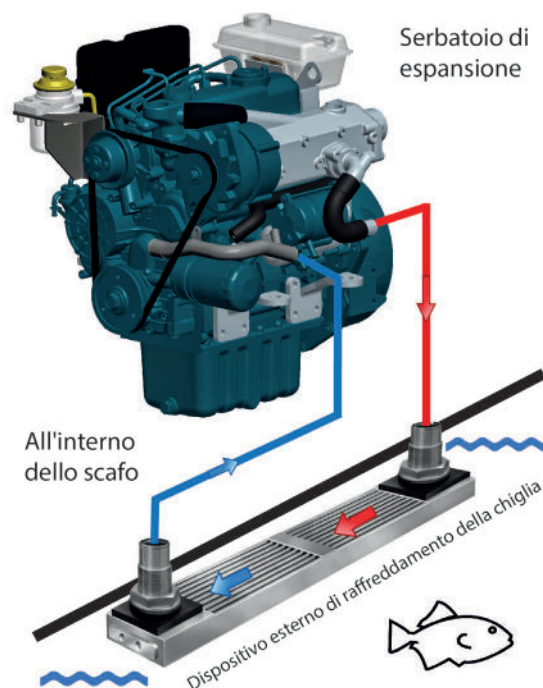
Principio del sistema di raffreddamento a chiglia sul motore
