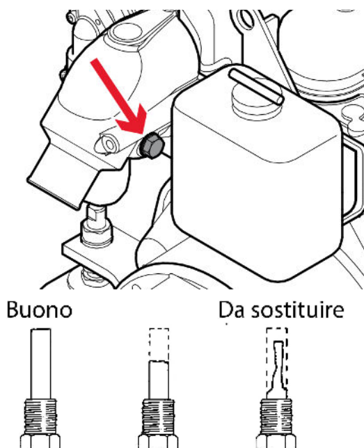
Anodi in zinco
