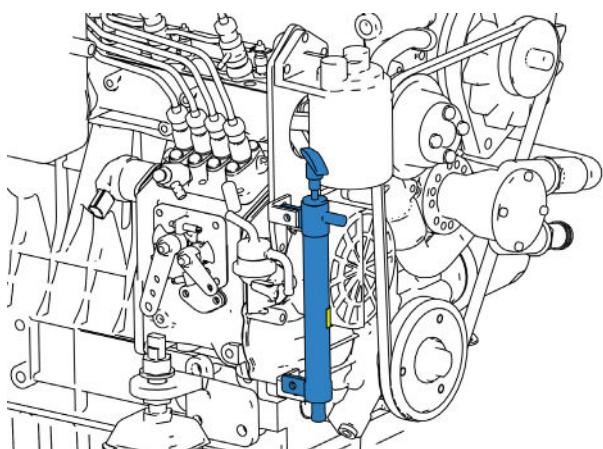
Nell'immagine sopra, la pompa manuale.
