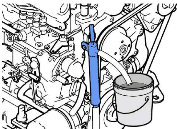
Visuale del drenaggio dell'olio dal motore
