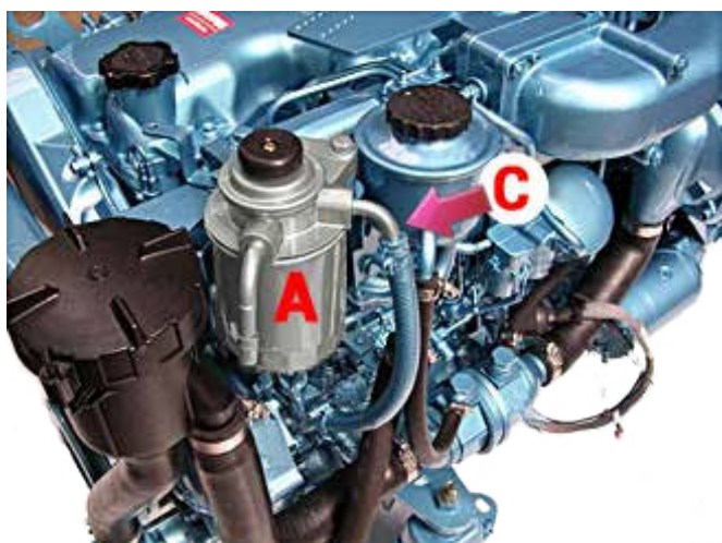
Ci-dessus : l'ensemble filtre à carburant
