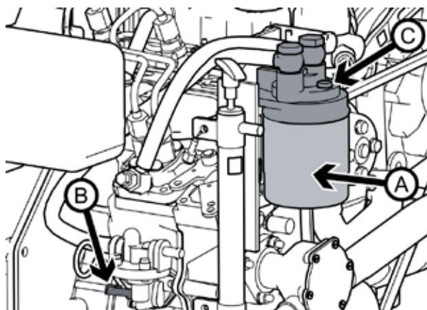
Ci-dessus : démontage du filtre carburant.
