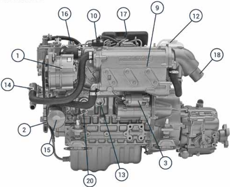
Figure 1: Vue avant du moteur N4.38
