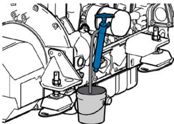
Vue de la vidange du moteur
